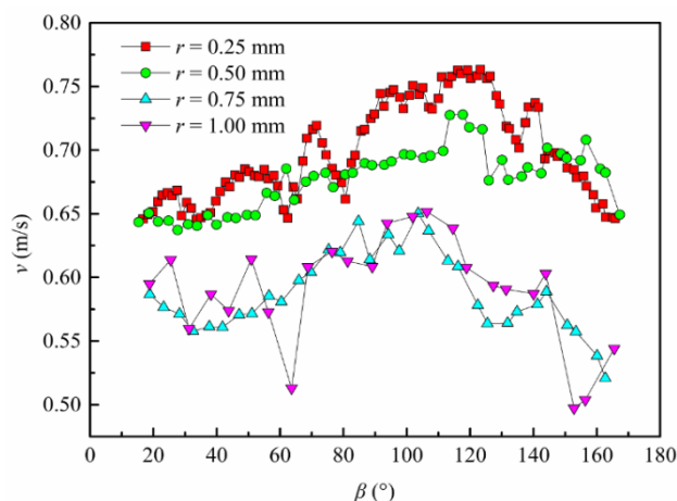
续图2.2 不同波纹半径下外波纹管周向液膜流动速度的变化
